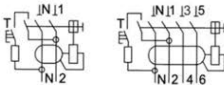
مدار الکتریکی کلید های محافظ جان مدل PFR
